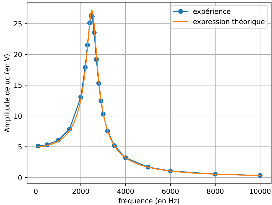
résonance en tension
