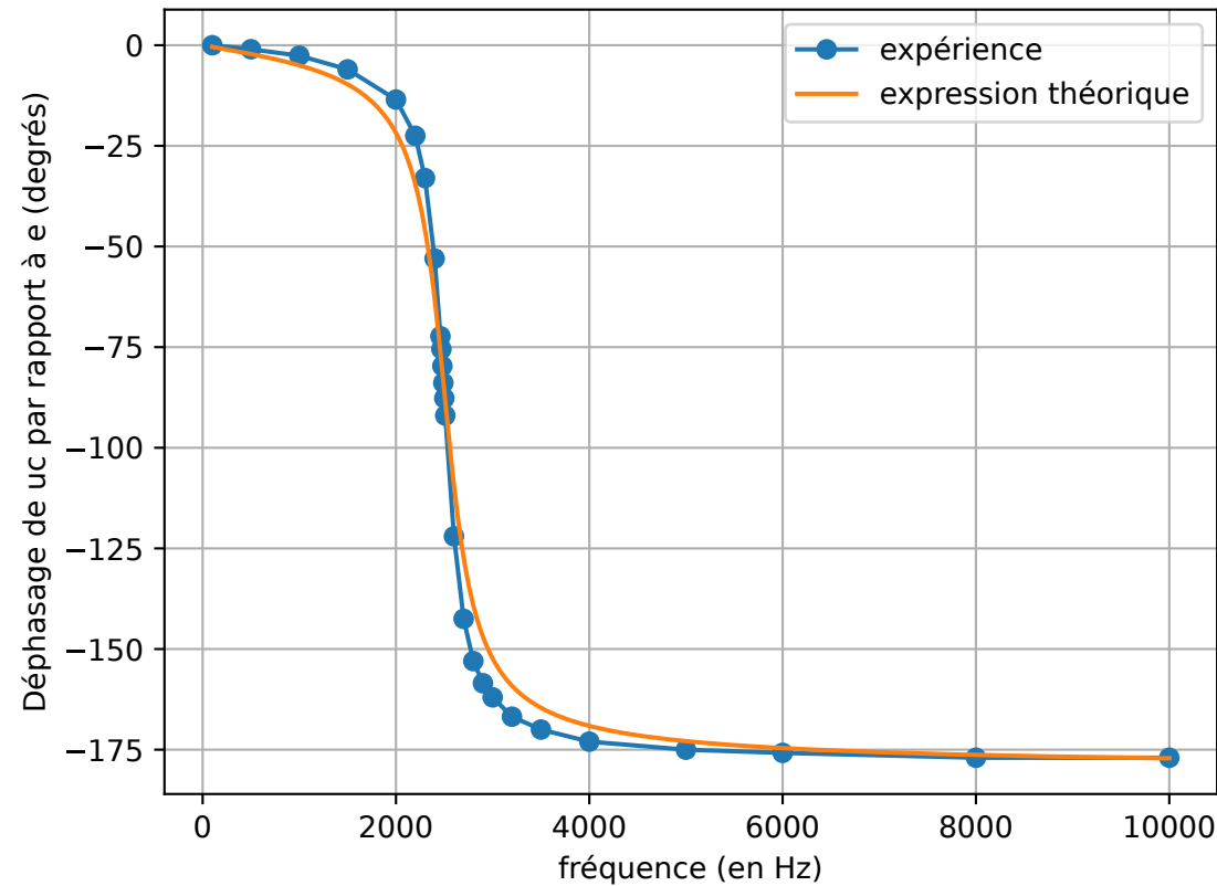
résonance en tension
