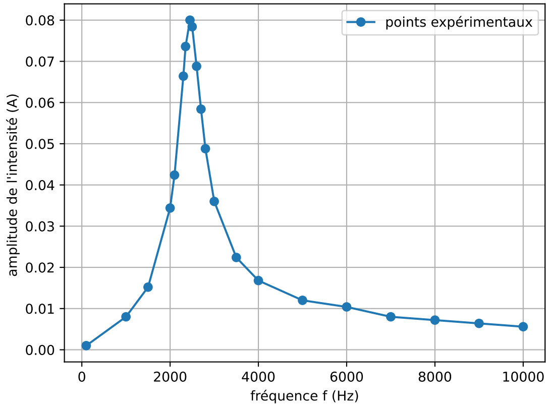
courbe de résonance, circuit RLC série
